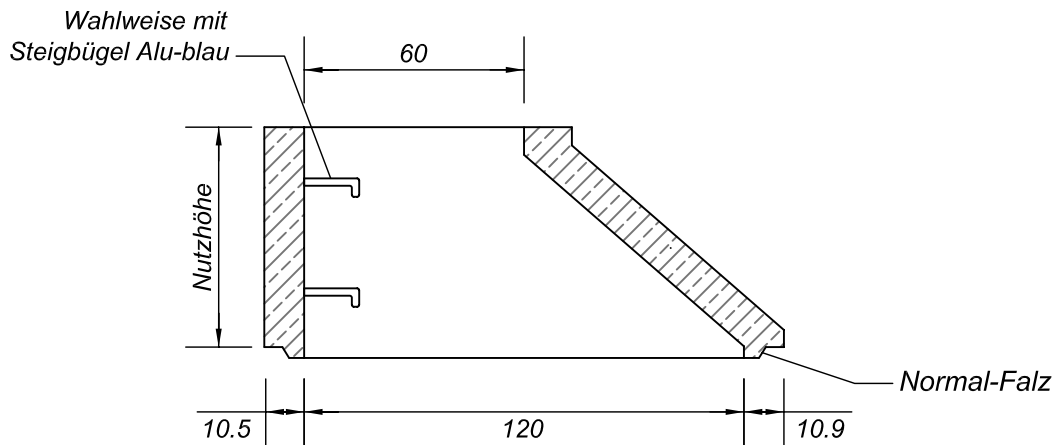
PIMA-Konus
